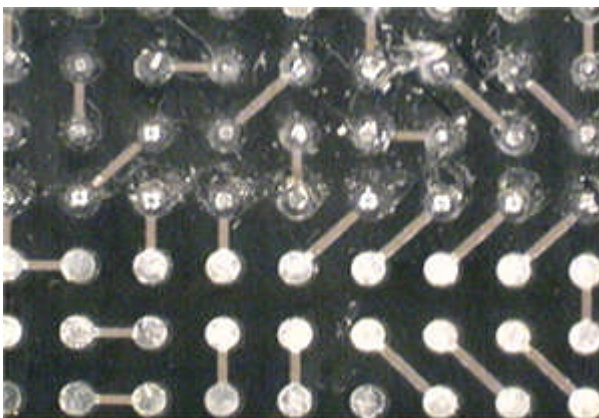
上側： はんだ除去前 下側： スカベンジング後
