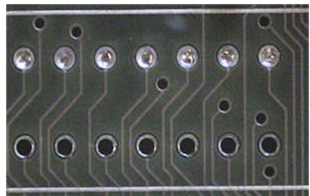
スルーホールのはんだ除去
