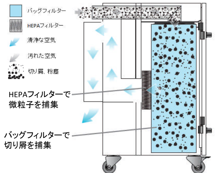
集塵フロー図
